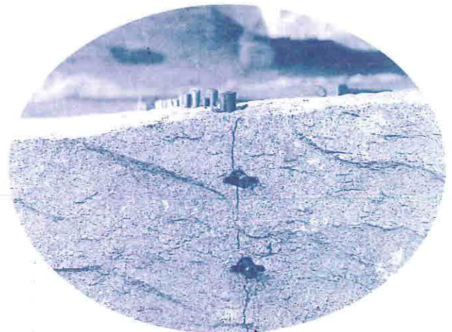
Tranchage d'un bloc de granit avec des coins de 22 x 115
