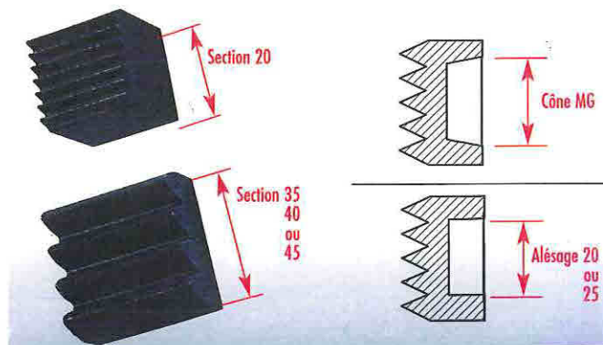
* Spéciales pour bouchardeuses mécaniques
